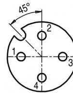
Polbild
