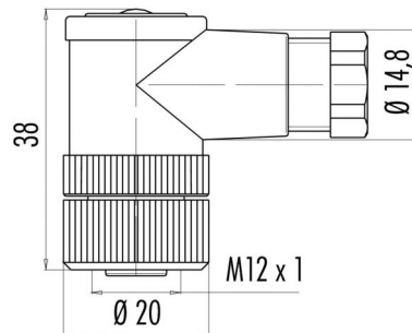
Maßzeichnung
