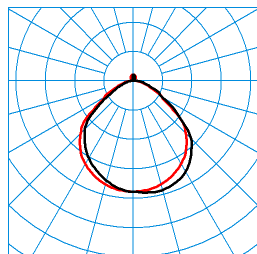
LuceoS D/H2-L CDP-A 5000-840 ETDD 03 (Pendant ZS/ZST+EB3) TX245968 DIN 5040: A40 UTE: 0,97 D + 0,03 T CEN Flux Code: 54 86 97 97 100 47 72 88 3
