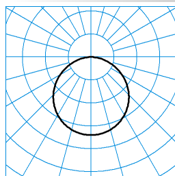
Skeo Circ MultiLC WD2 1G1Y ETDD (ww) ■ C0 - C180 TX059430 UGR I = 22,8 UGR q = 22,8 DIN 5040: A40 UTE: 1,00 E CEN Flux Code: 46 78 96 100 100
