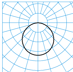
Skeo Circ MultiLC WD2 1G1Y ETDD (cw) ■ C0 - C180 TX278652 UGR I = 22,8 UGR q = 22,8 DIN 5040: A40 UTE: 1,00 E CEN Flux Code: 46 78 96 100 100
