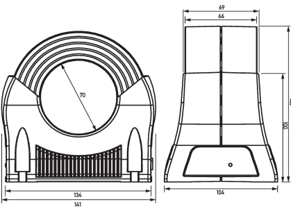
Maßzeichnung Gruppenansicht
