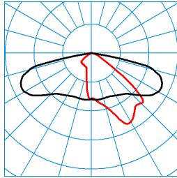
Cuvia 40-AB2L-LRA/1350-740 2G1S TX046949
