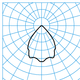
InperiaLP C05 HR22 IP 1800-830 03 + ZN-PC TX052464 ■ C0 - C180
