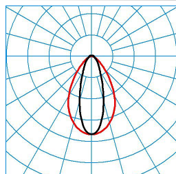
ELINE PN100 840 L225 1 50
