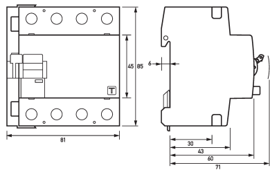
Maßzeichnung Gruppenansicht
