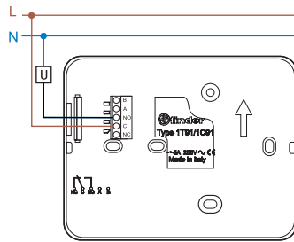
Anschlussbild
