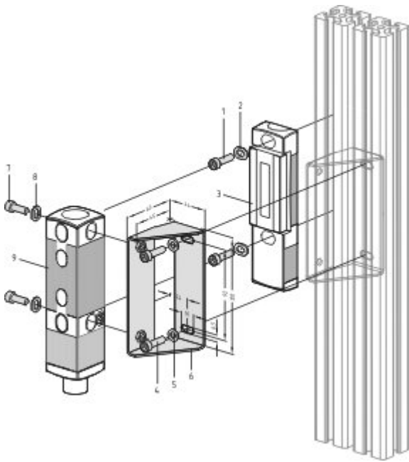
Produktgrafik (Explosionszeichnung)
