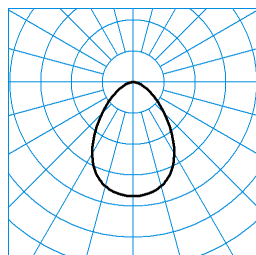
InperlaLP C05 BR22 1000-840 03 + DA-M 03 TX041236 ■ C0 - C180
