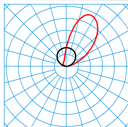
Altigo G2 120 WO GS AM15L/700-840 + G2 VE IP66 24V DC 120W TX113590
