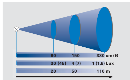
Reichweiten-Diagramm SEB 10
