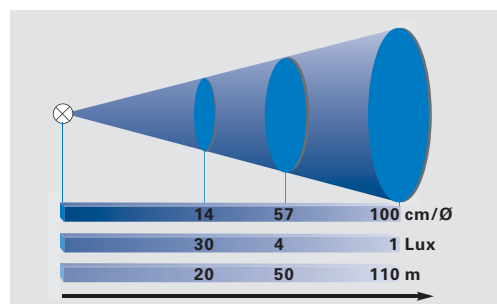
Reichweiten-Diagramm SEB 9 / 8
