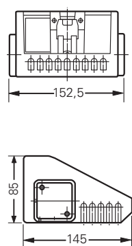
Maßzeichnung Wandhalter SW
