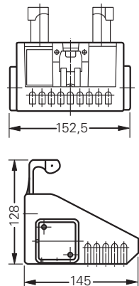
Maßzeichnung Kfz-Halter 90
