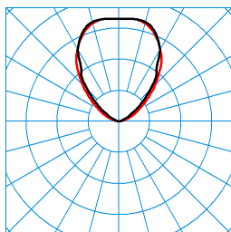
Altigo G2 120 WO GS SE7L/1300-830 1G1P + G2 VE IP66 24V DC 80W TX113683
