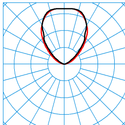
Altigo G2 120 WO GS SE7L/1300-830 1G1P + G2 VE IP66 24V DC 240W TX113681
