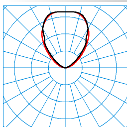
Altigo G2 120 WO GS SE7L/1300-830 1G1P + G2 VE IP66 24V DC 120W TX113680
