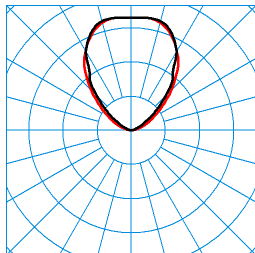
Altigo G2 120 WO GS SE7L/1300-830 1G1P + G2 VE IP66 24V DC 30W TX113682
