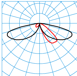
LTX KT-AB2L-LRA/15/18/26-740 4G1 (1800 lm) TX084045
