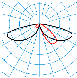
LTX KT-AB2L-LRA/15/18/26-740 4G1 (1500 lm) TX084044
