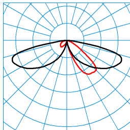
LTX KT-AB2L-LRA/15/18/26-740 4G1 (2600 lm) TX084046
