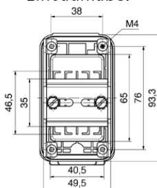
Einbaumaße:
