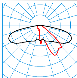
Publisca P2-AB2L-LRA/2600-740 3G1S TX047789
