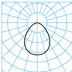
InperiaL G2 C07 BR22 2700-830 03 + DA-M 03 TX052913 ■ C0 - C180
