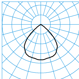
InperiaL G2 C07 BR22 2700-830 03 + DA 03 TX052912 ■ C0 - C180
