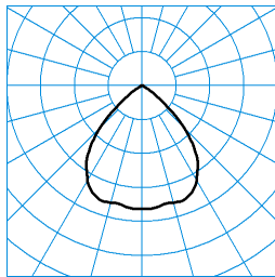
InperiaL G2 C07 BR22 2700-830 03 + RD-PC TX052914 ■ C0 - C180
