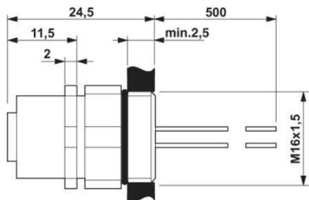
M12-Einbaubuchse, positionierbar
