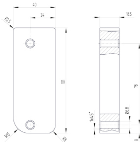
Maßzeichnung (Sonstige)
