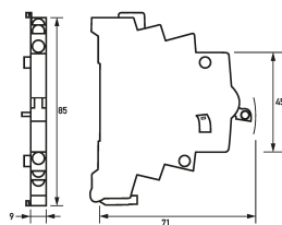
Maßzeichnung Gruppenansicht
