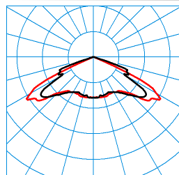
E-Line Fi L-SLB 230V CEAG L37 05 TX122096
