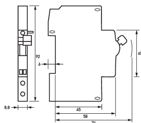
Maßzeichnung Gruppenansicht
