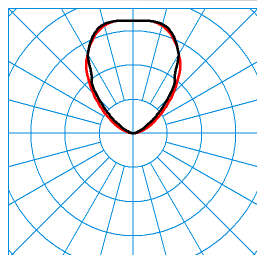
Altigo G2 60 WO GS SE7L/700-830 1G1P + G2 VE IP66 24V DC 120W TX113692
