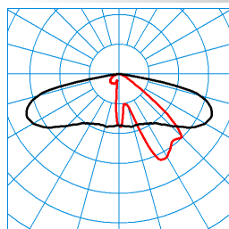
Publisca P2-AB2L-LRA/1650-730 2G1S TX047778
