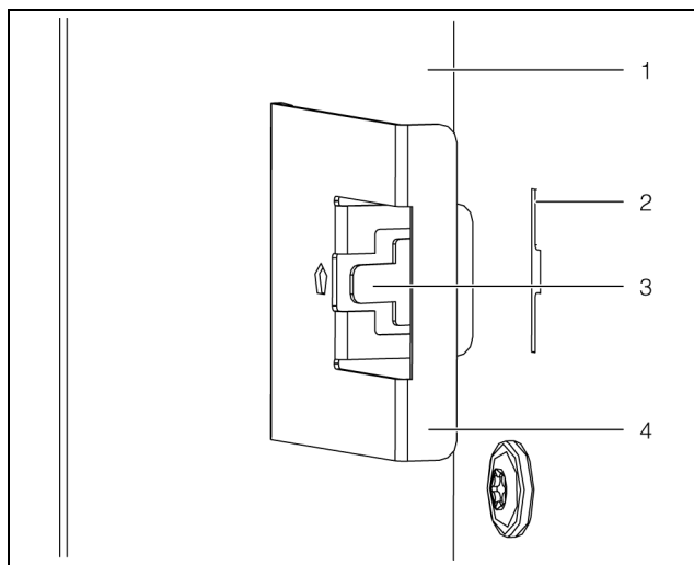
Imagen 34: Retirar los bornes elásticos
