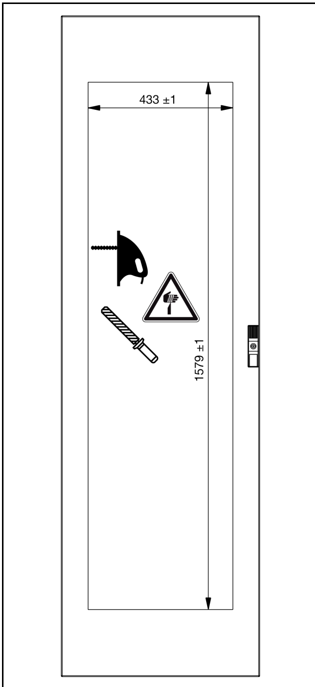
Imagen 38: Escotadura de montaje
