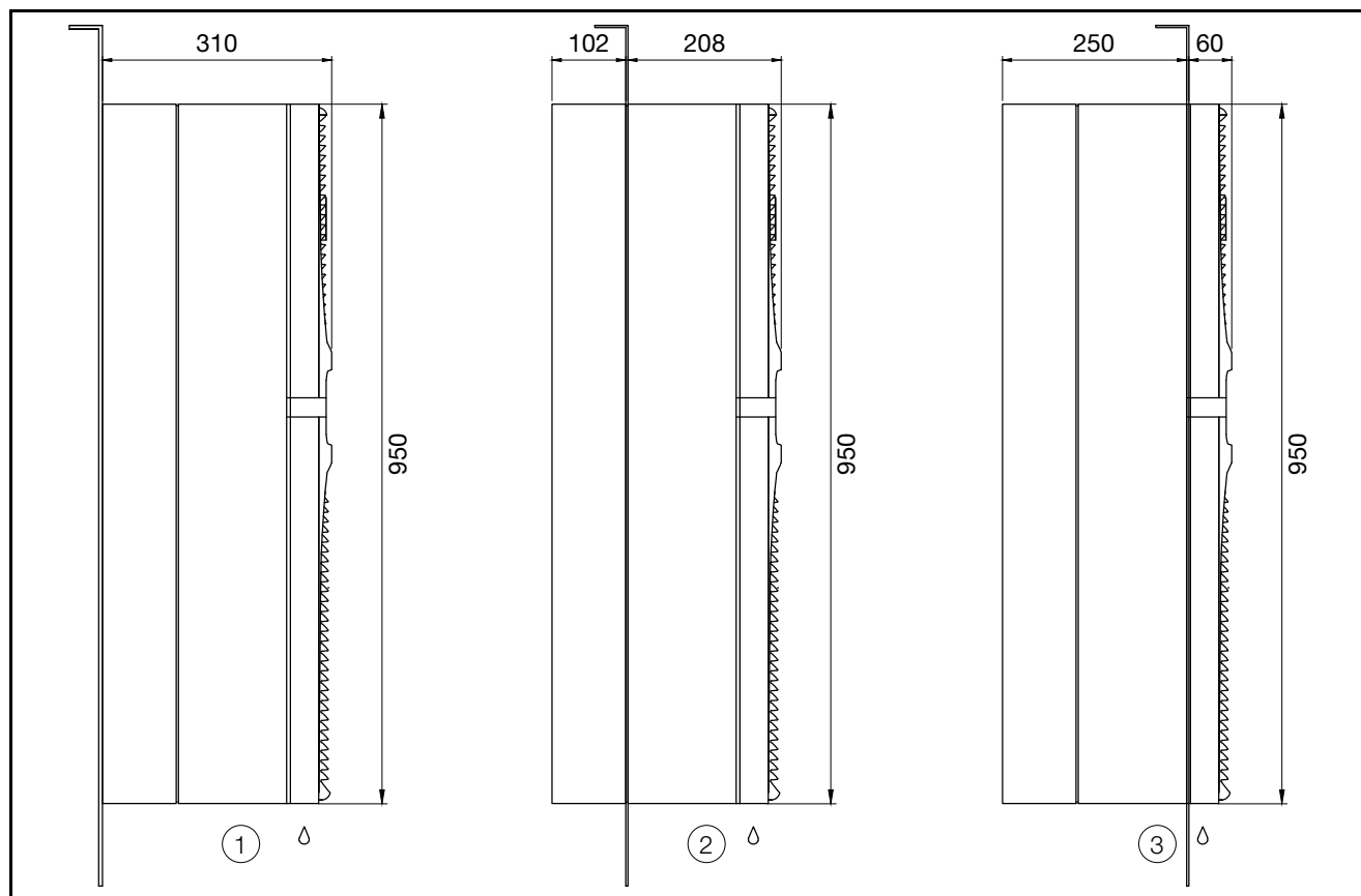
Imagen 40: Dimensiones SK 3185830
