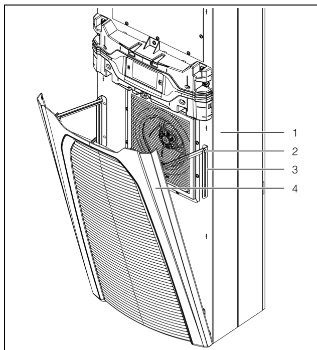
Imagen 29: Fijaciones en el mecanismo abatible (imagen de ejemplo)
