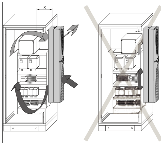
Imagen 5: No orientar nunca el caudal de aire frío hacia componentes activos (imagen de ejemplo)
