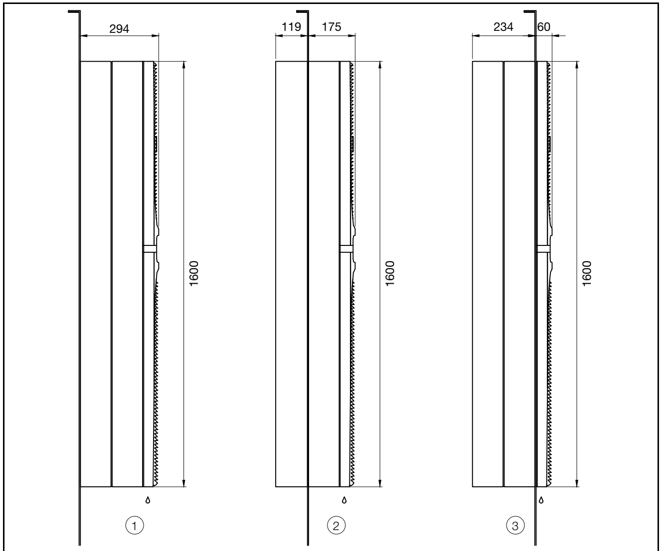
Imagen 41: Dimensiones SK 3186930 y SK 3187930
