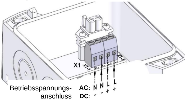
PY L-S mit Einzelfarben-LED
