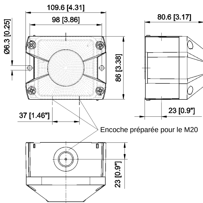
Schéma de perçage de l'intérieur du boîtier
