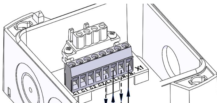
РУ L-S с многоцветным СИД
