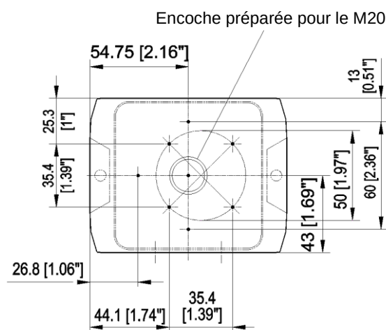
Schéma de perçage de l'intérieur du boîtier
