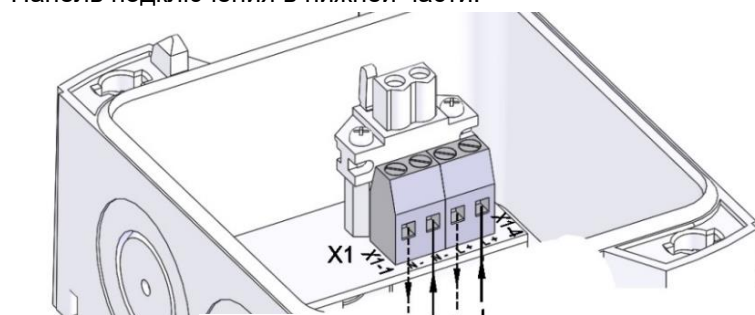
РУ L-S с одноцветным СИД
