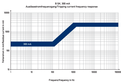
Kennlinie B SK 300 mA
