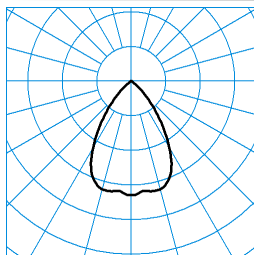
InperiaL G2 C07 HR22 3800-830 01 ■ C0 - C180 TX053097
