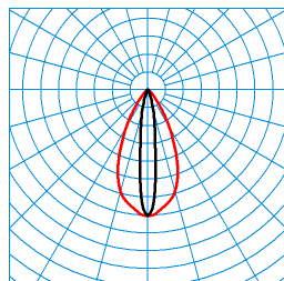
Altigo G2 10 SE6L/300-830 1G1P + G2 VE IP66 24V DC 30W TX113662 ■ C0 - C180 ■ C90 - C270 UGR I = 18,3 UGR q = 9,9 DIN 5040: A70 UTE: 1,00 A CEN Flux Code: 93 98 99 100 100
