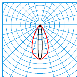
Altigo G2 10 SE6L/300-830 1G1P + G2 VE IP66 24V DC 240W TX113661 ■ C0 - C180 ■ C90 - C270 UGR I = 18,3 UGR q = 9,9 DIN 5040: A70 UTE: 1,00 A CEN Flux Code: 93 98 99 100 100
