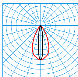
Altigo G2 10 SE6L/300-830 1G1P + VE IP66 24V DC 130W TX120370 ■ C0 - C180 ■ C90 - C270 UGR I = 18,3 UGR q = 9,9 DIN 5040: A70 UTE: 1,00 A CEN Flux Code: 93 98 99 100 100
