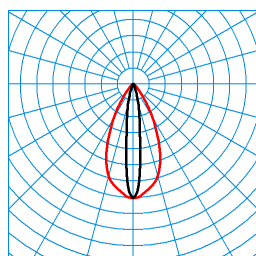
Altigo G2 10 SE6L/300-830 1G1P + G2 VE IP66 24V DC 80W TX113663 ■ C0 - C180 ■ C90 - C270 UGR I = 18,3 UGR q = 9,9 DIN 5040: A70 UTE: 1,00 A CEN Flux Code: 93 98 99 100 100
