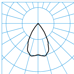
InperiaLP C05 HR22 2700-830 03 TX373869 ■ C0 - C180
