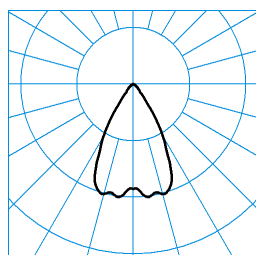
InperlaLP C05 HR22 2700-830 03 + RD-PC ■ C0 - C180 TX373864
