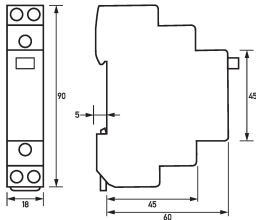
Maßzeichnung Gruppenansicht
