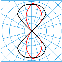
Skeo Q-W2 GT AB19R-AB19R/1600-840 TX084369 DIN 5040: C64 UTE: 0,50 B + 0,50 T CEN Flux Code: 81 99 100 50 100 81 99 100 50
