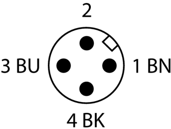
Schaltplan
