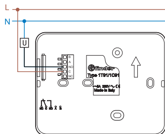
Anschlussbild
