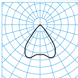
InperiaL G2 C07 HR19 2700-830 03 ■ C0 - C180 TX053031
