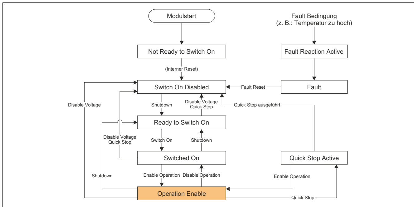
Abbildung 4: State Machine - Flussdiagramm
