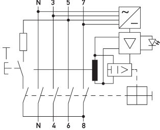
Anschlusschema
