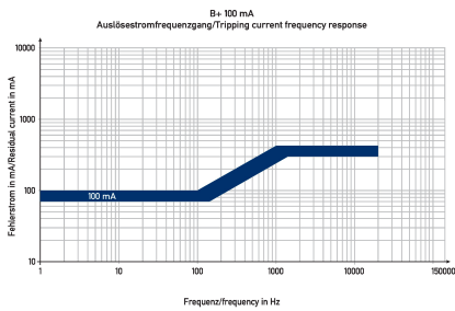
Kennlinie B+ 100 mA
