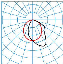
Arimo M57 RAV LED4500-840 ETDD 01 TX277664
