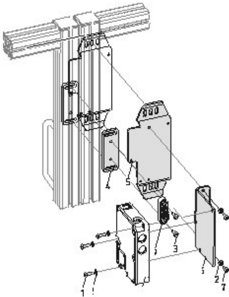
Produktgrafik (Explosionszeichnung)
