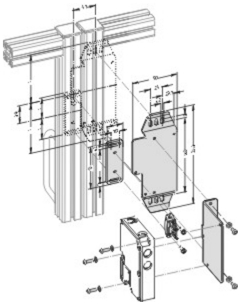
Maßzeichnung (Sonstige)
