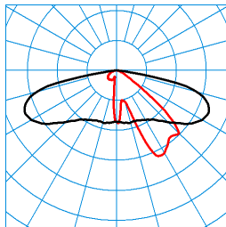
Publisca P1-AB2L-LR/2200-730 3G1S TX047519
