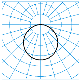
Skeo Circ MultiLC WD2 1G1Y ET +HFS E3 (ww) ■ C0 - C180 TX195237 UGR I = 22,8 UGR q = 22,8 DIN 5040: A40 UTE: 1,00 E CEN Flux Code: 46 78 96 100 100
