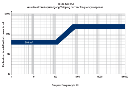
Kennlinie B SK 500 mA
