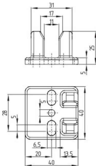
Maßzeichnung (Grundgerät)
