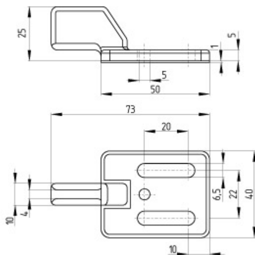
Maßzeichnung (Grundgerät)
