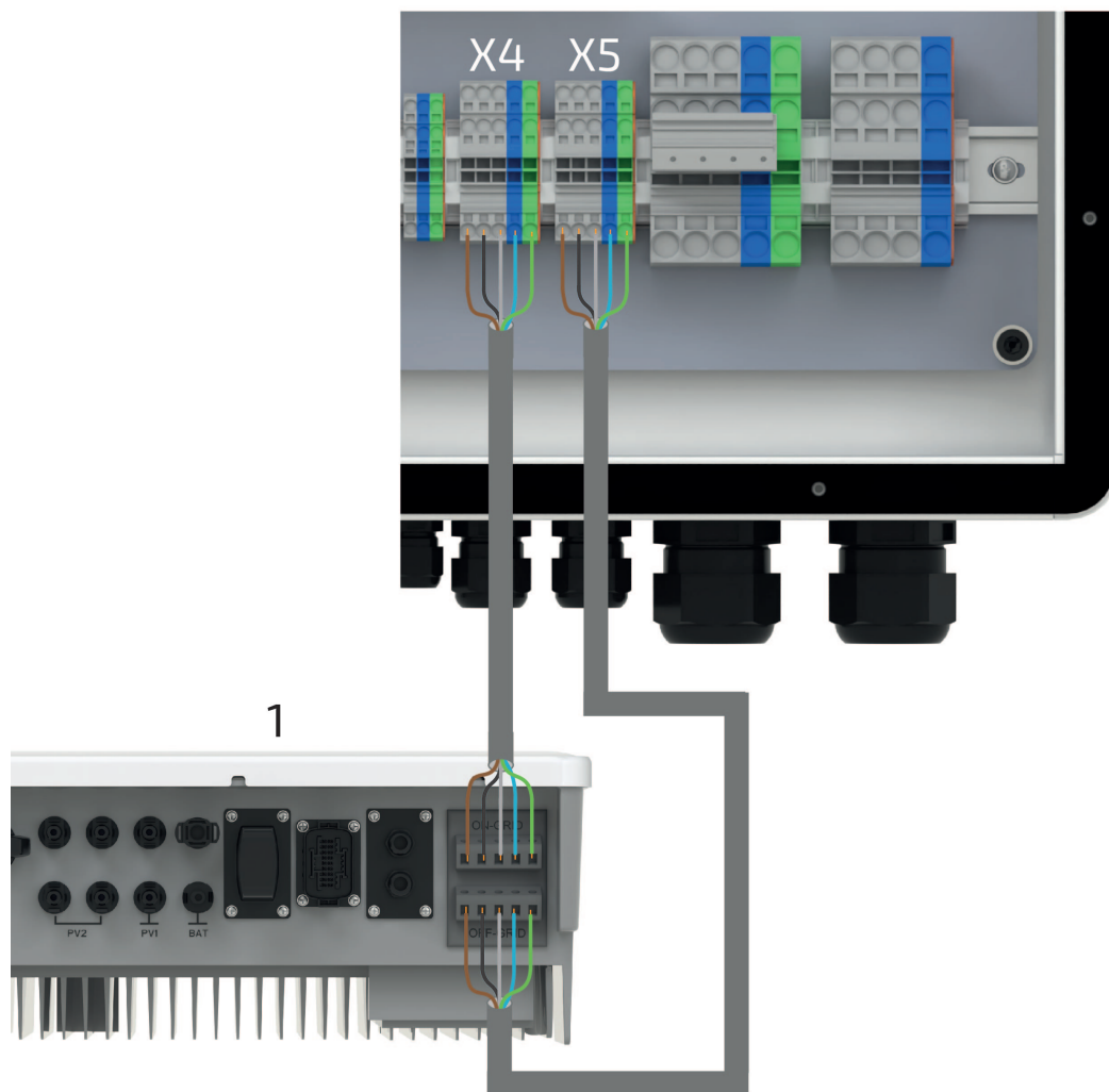
Abbildung 8. AC-Anschluss Wechselrichter
