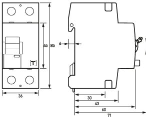
Maßzeichnung Gruppenansicht
