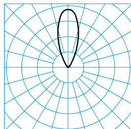
Altigo G2 120 WO RB17L/3800-830 1G1P + G2 VE IP66 24V DC 30W TX113958 ■ C0 - C180
