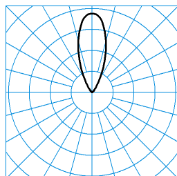
Altigo G2 120 WO RB17L/3800-830 1G1P + G2 VE IP66 24V DC 240W TX113944 ■ C0 - C180
