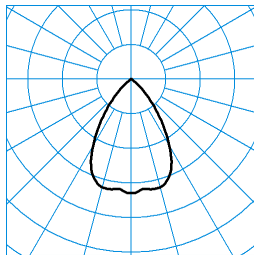
InperiaL G2 C07 BR25 4700-830 01 ■ C0 - C180 TX373464
