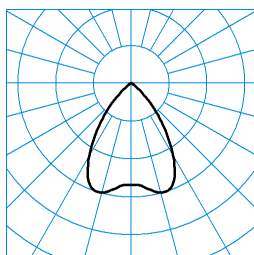
InperiaL G2 C07 BR25 4700-830 01 + DA 01 ■ C0 - C180 TX373462
