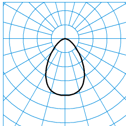
InperiaL G2 C07 BR25 4700-830 01 + DA-M 01 ■ C0 - C180 TX373461
