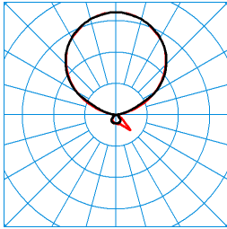
LuceoS S G2 PAW-IL 150-830 ETDS 01 TX299600
