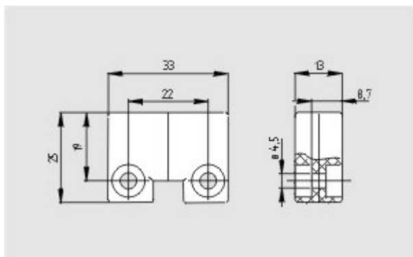
Maßzeichnung (Sonstige)
